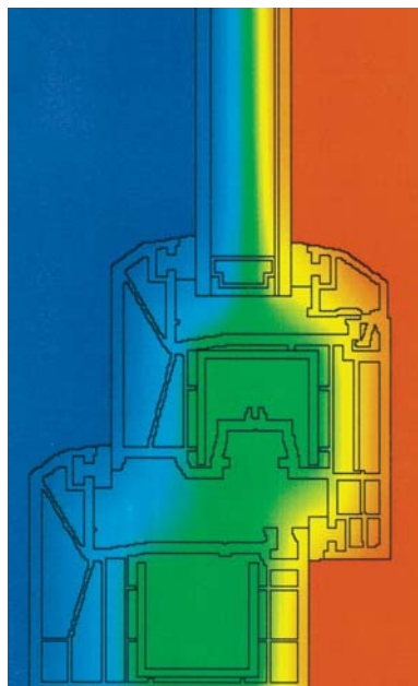
Wärmedämmung: Das Temperaturbild zeigt den optimierten Verlauf der Isothermenkurven.
